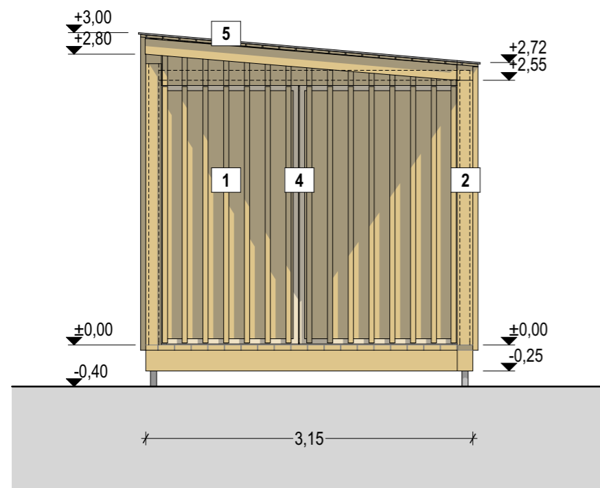
DNY Homlokzat m 1:50
