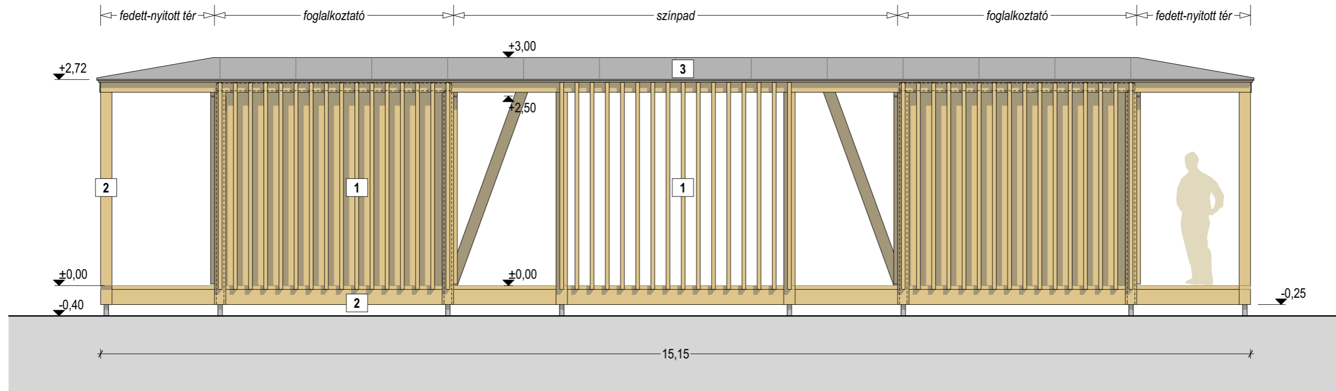
DK Homlokzat m 1:50
